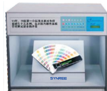
SR-732標準光源箱 SUPER DAYLIGHT
